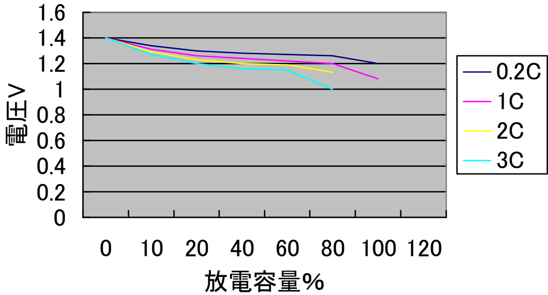
放電曲線
