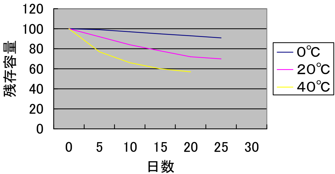
温度別自己放電
