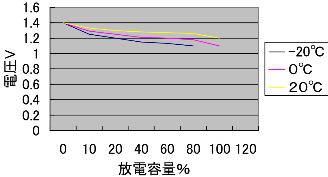
温度変化による放電特性(0.2C,A)
