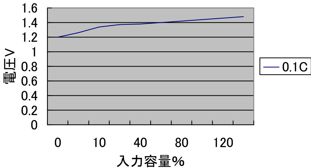
充電特性(20°C)
